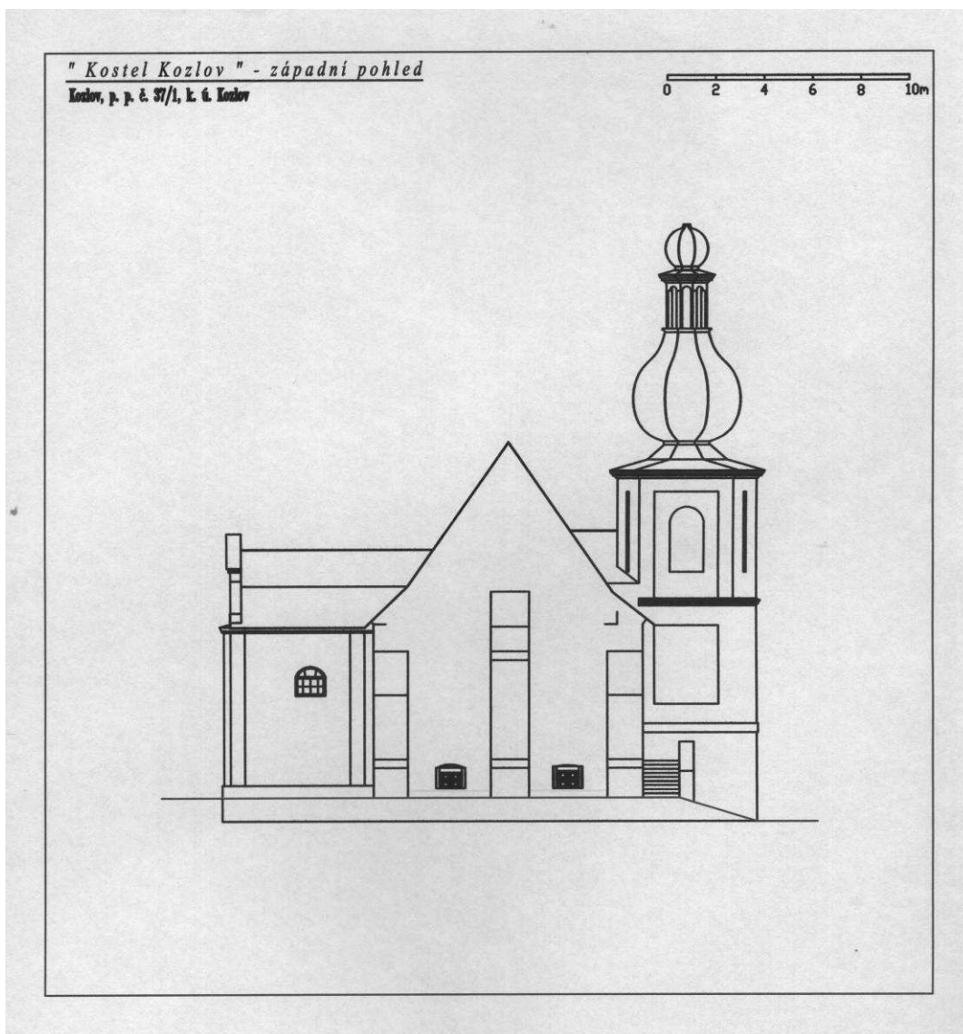
Nárys kostela – západní strana
