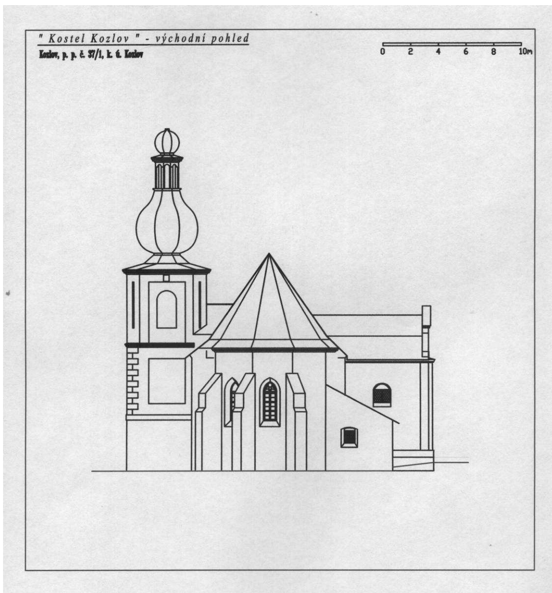
Nárys kostela – východní strana
